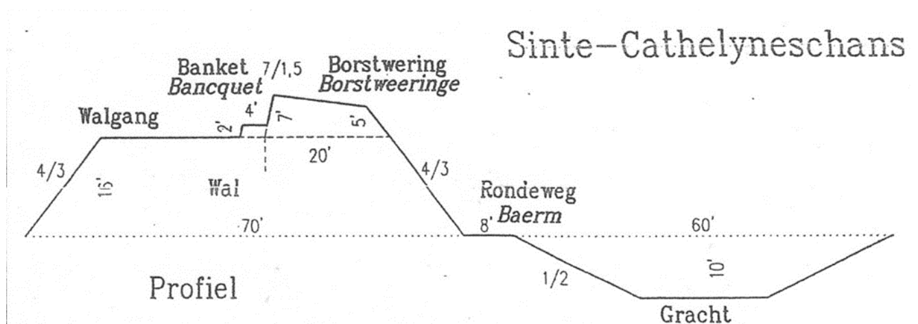
Figuur 4 – Voorbeeld van een profiel van een aarden fort uit de 16 de eeuw. Het gaat om het profiel volgens het bestek van de Sinte-Cathelyneschans bij Koewacht (NL). Afmetingen in voet (één geometrische voet meet 0,307 - - (ARA Brugge)
